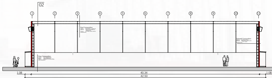
SECTION 01
